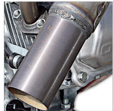
passender Katalysator für Benzin-Motor
