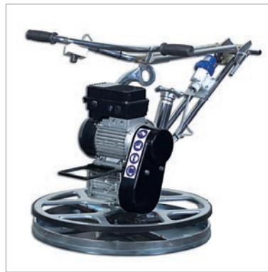
MOSKITO SG Elektro
